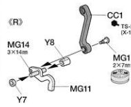
《ゲートロック》 Gate locks Klappenverriegelung Verrous de battant articulé
