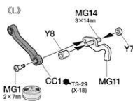
MG11 荷台ゲートロック Gate lock Klappenverriegelung Verrou de battant
